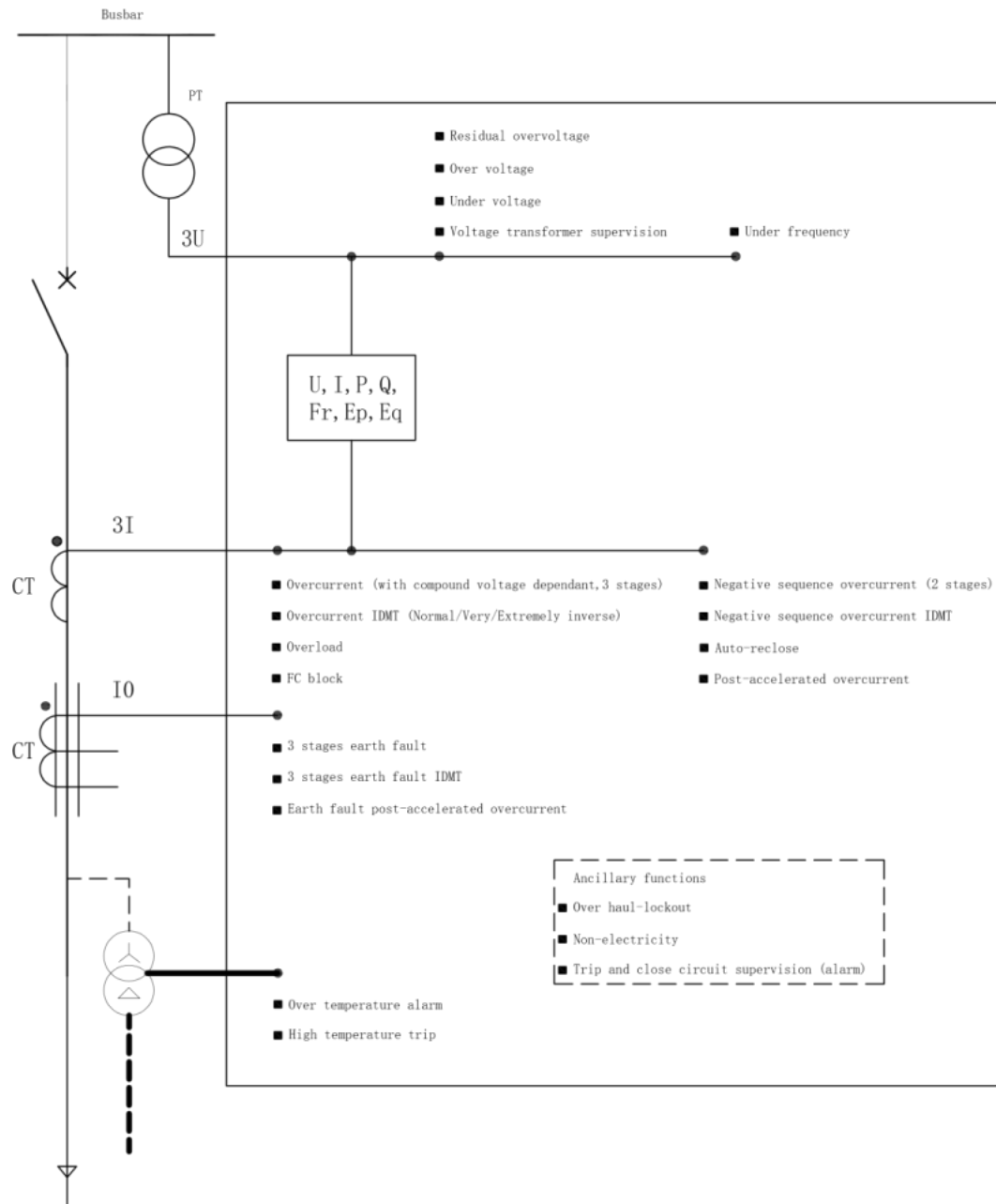
Fig. 5.3 VKRV-VI function diagram
